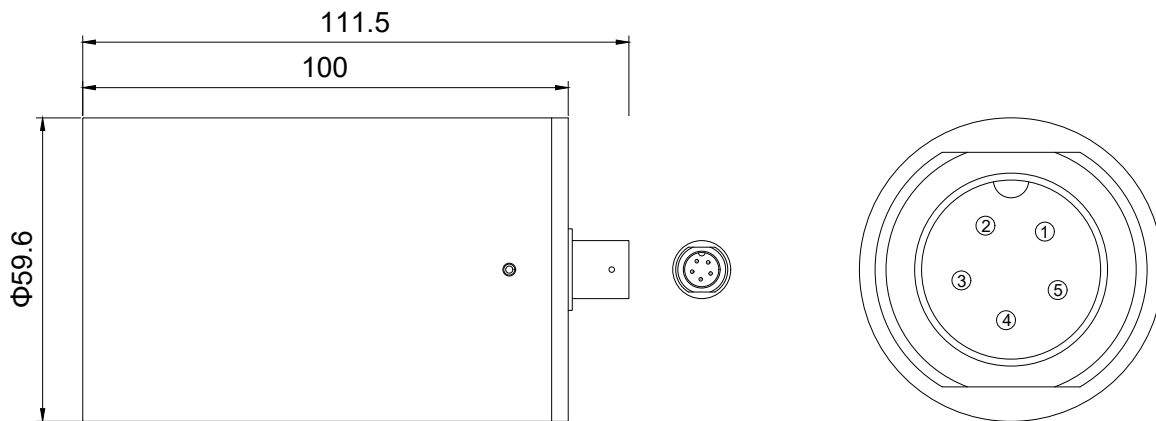
单位：mm 2英寸探测器
